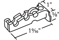
#018-24 Die Cast Steel 9/16" Dia. Roller
