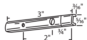
#030-304 Universal Pivot Bar
