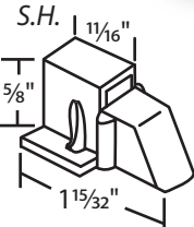
#02-0562 Top Bracket S.H.
