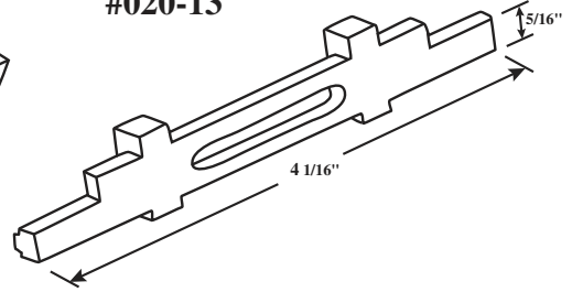
#020-15LH #020-15RH RH Shown
