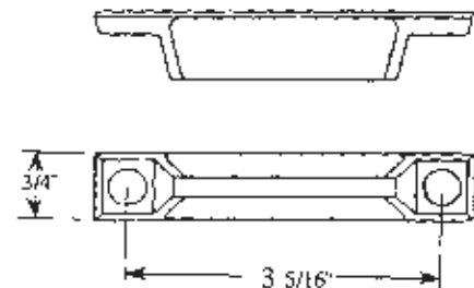
#014-24-XX Die Cast Specify Color
