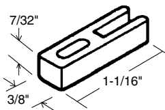
Sliding Screen Door Guide
