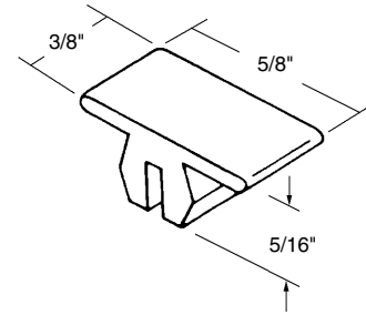
Sliding Screen Door Top Guide
