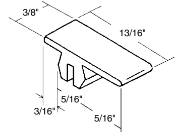
Sliding Screen Door Top Guide
