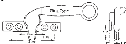
#04-55 RH Shown #04-56 LH
